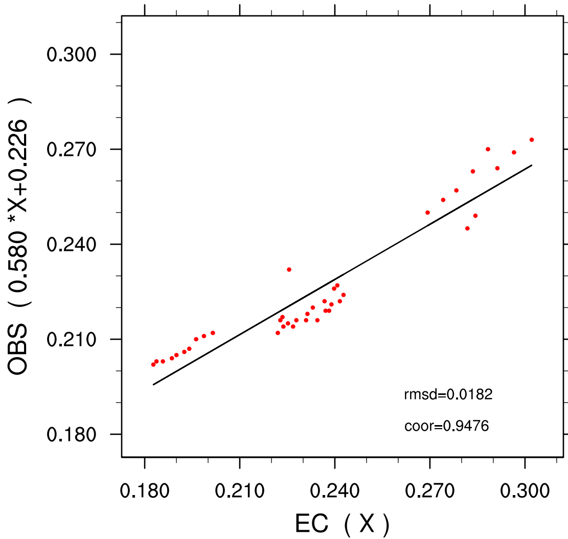
Banatski_Karlovac EC-OBS JUL dec=1
