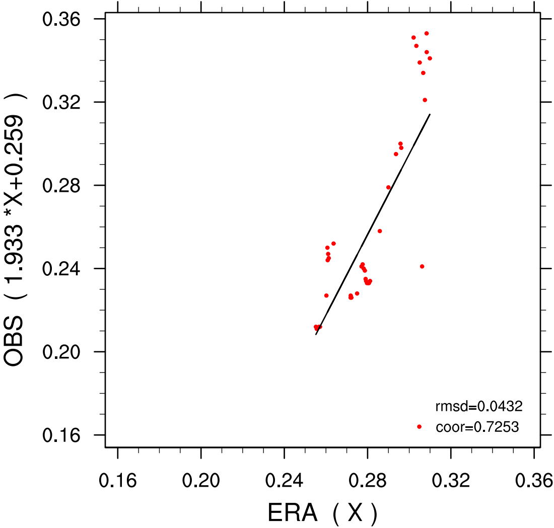
Beograd_Vracar ERA-OBS DEC dec=2
