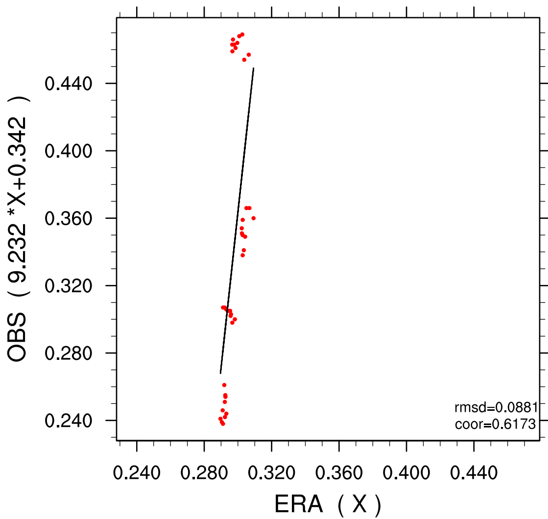
Beograd_Vracar ERA-OBS FEB dec=1
