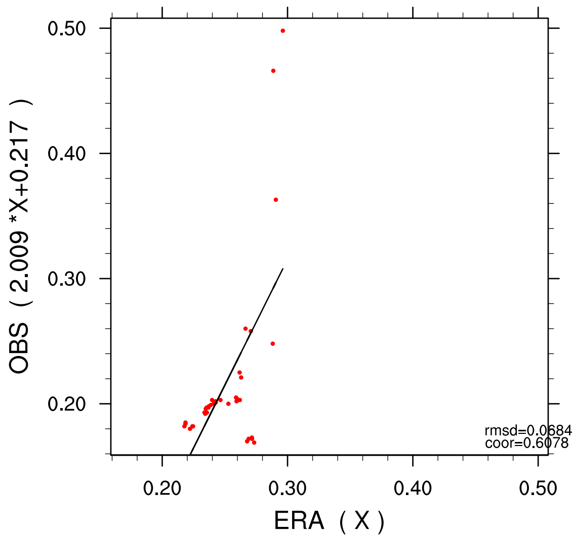
Beograd_Vracar ERA-OBS JUL dec=3
