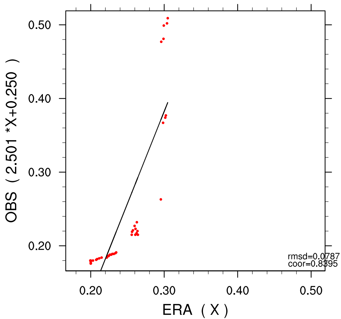
Beograd_Vracar ERA-OBS AUG dec=1
