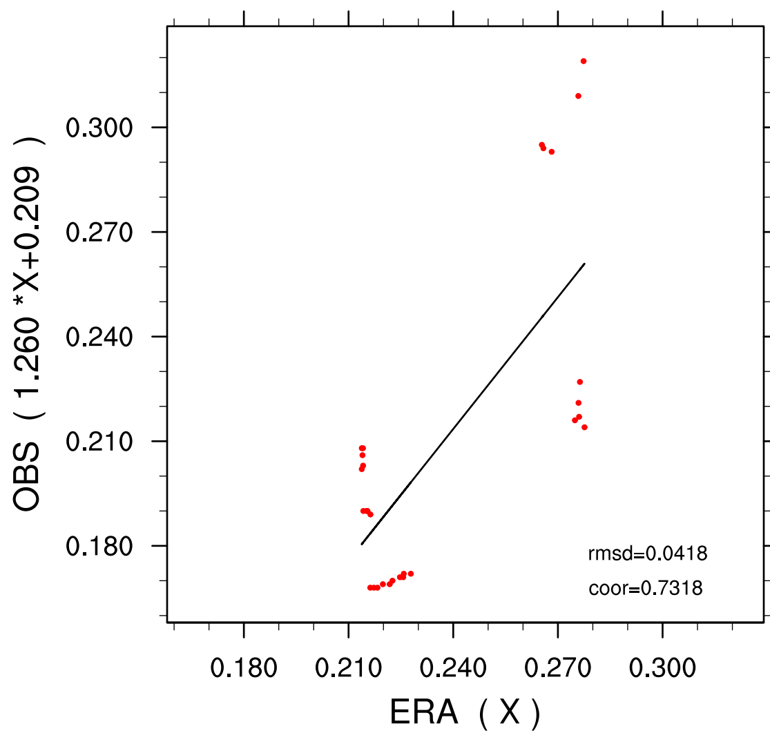
Beograd_Vracar ERA-OBS SEP dec=1
