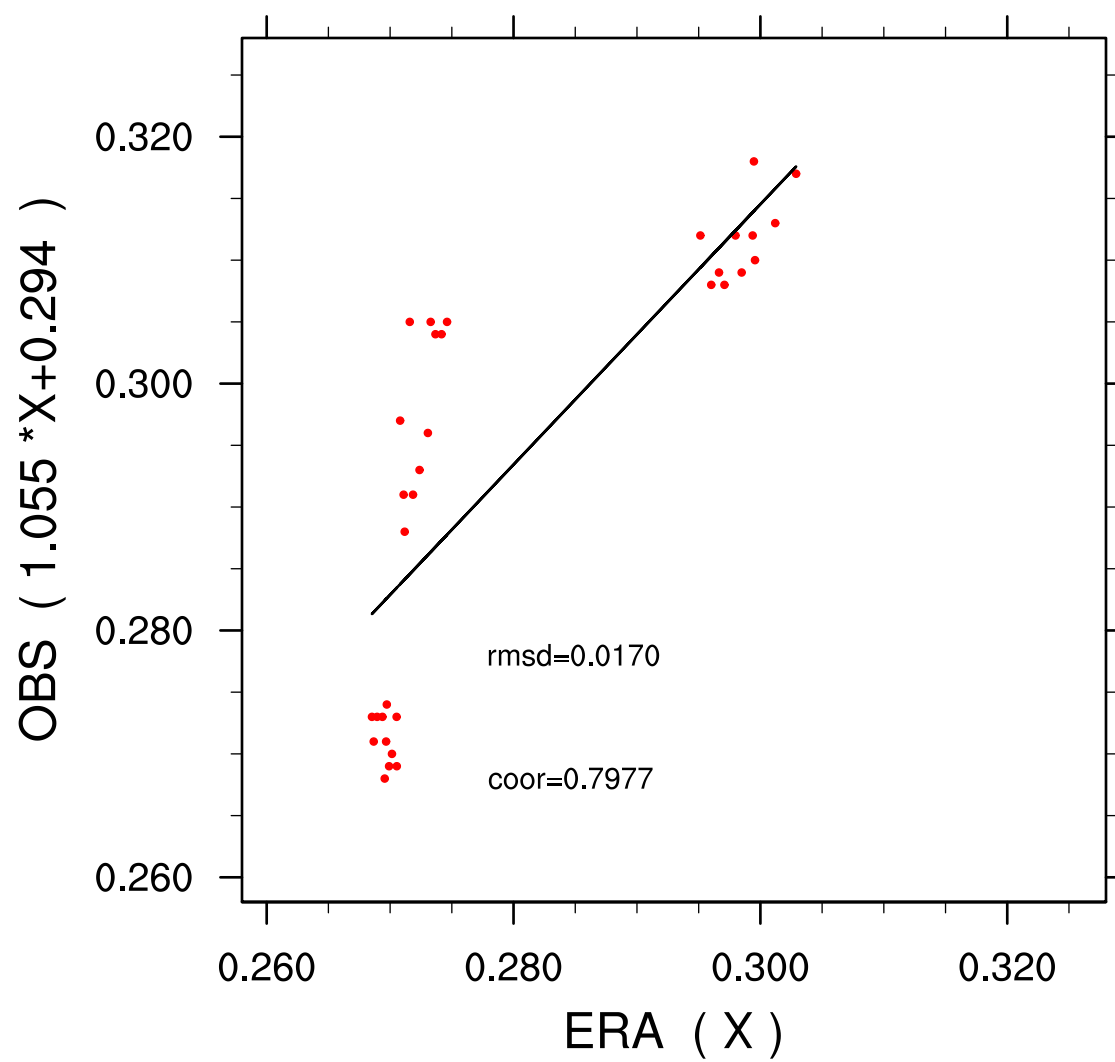
Leskovac ERA-OBS DEC dec=3
