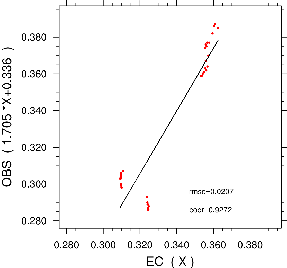
Smederevska_Palanka EC-OBS FEB dec=1
