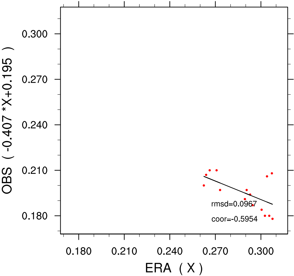
Smederevska_Palanka ERA-OBS JUL dec=2
