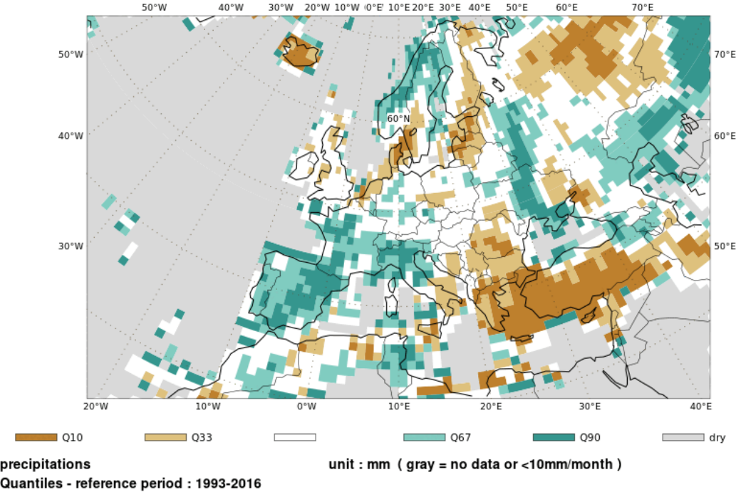
Fig. 5.2: Quantiles of monthly precipitation totals for October 2024. Source : Météo France, http://seasonal.meteo.fr/content/suivi-clim-cartes-ref93-16 , data source : GPCP
